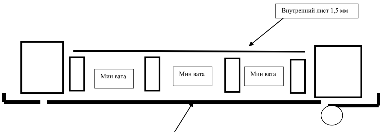
сечение двери
